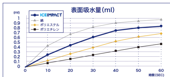
JIS L1907-2010 改良ラローズ法
